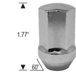
DODGE OEM LUG NUT LONG
