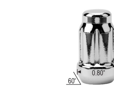
SPLINE LUG NUT 6PT
