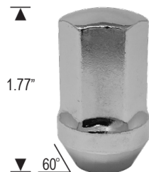
DODGE OEM LUG NUT LONG
