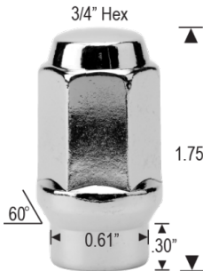
LONG ET BULGE LUG
