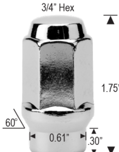
LONG ET BULGE LUG
