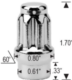
ET SPLINE 6PT
